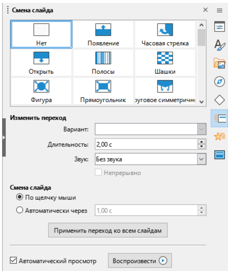
Рисунок 127 – Панель Смена слайда
