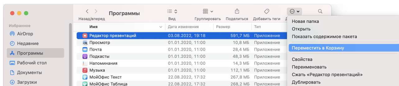
Рисунок 17 – Кнопка Действие
