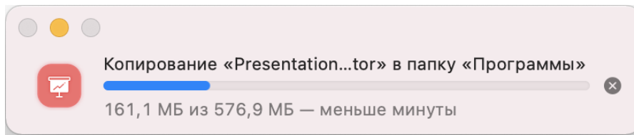
Рисунок 8 – Копирование приложения
