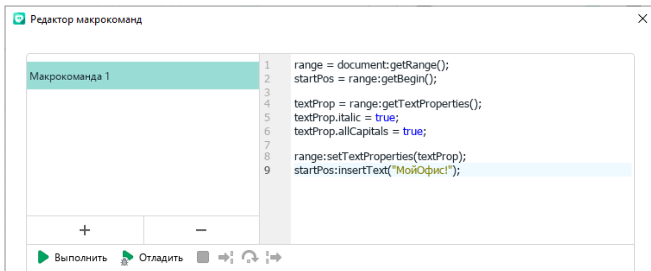
Рисунок 279 – Ввод текста макроккоманды
