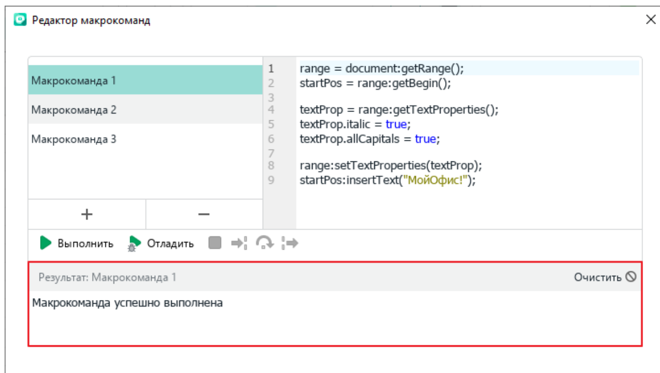
Рисунок 284 – Результат выполнения макроккоманды
