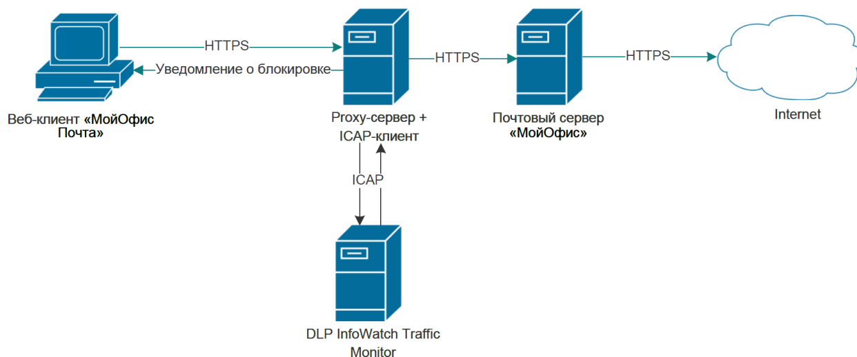
Рисунок 4. Установка DLP Infowatch traffic monitor “в разрыв” (режим блокировки)
