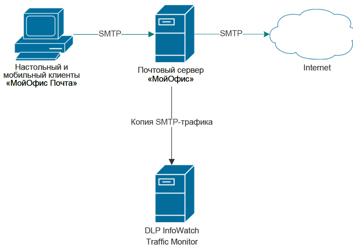
Рисунок 3. Установка DLP Infowatch Traffic Monitor в разрыв (режим “скрытая копия”)
