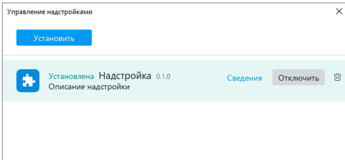
Рисунок 332 – Строка надстройки
