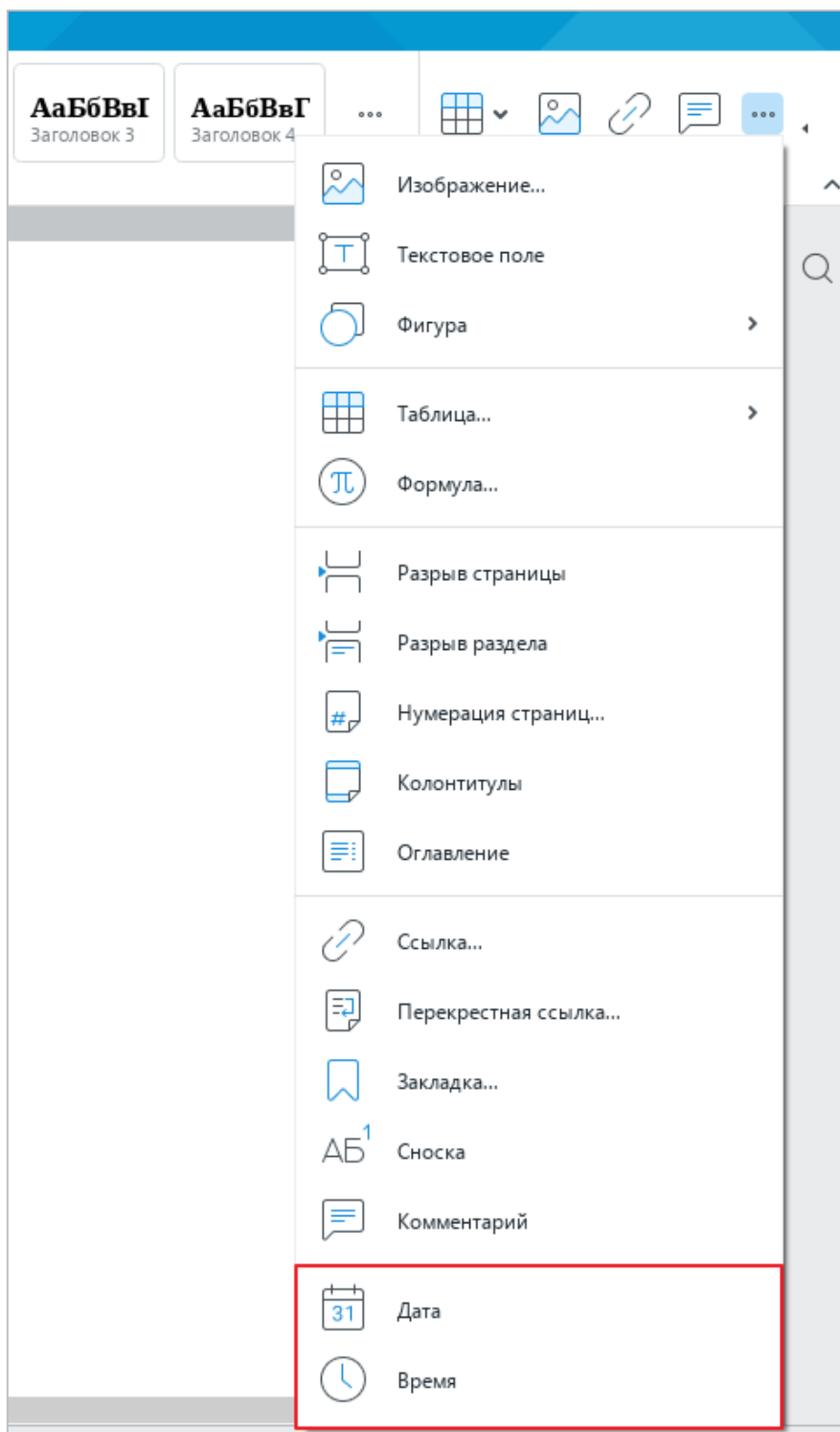
Рисунок 129 – Панель вставки
