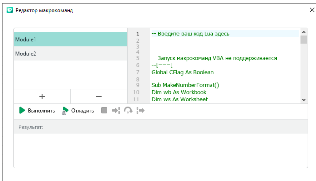
Рисунок 357 – Окно Редактор макрокоманд
