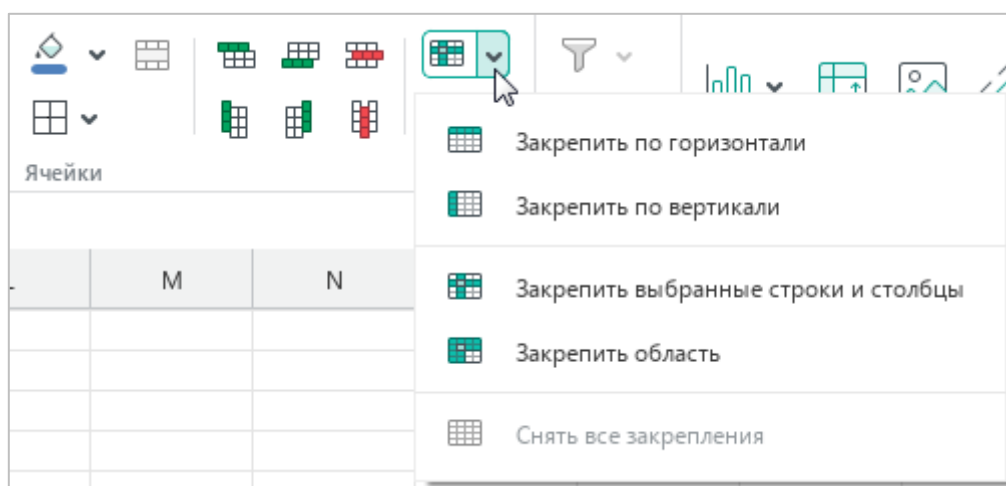
Рисунок 50 – Управление закрепленными элементами
