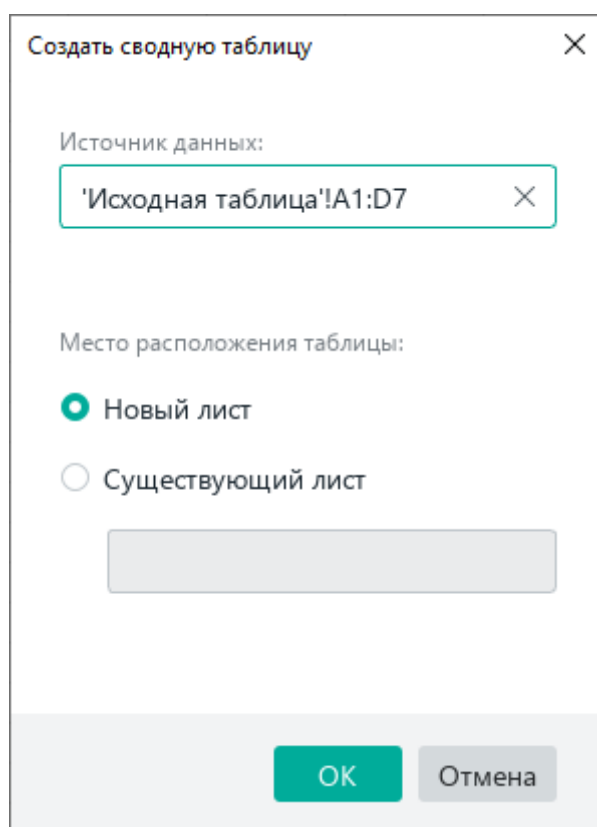
Рисунок 231 – Окно Создать сводную таблицу
