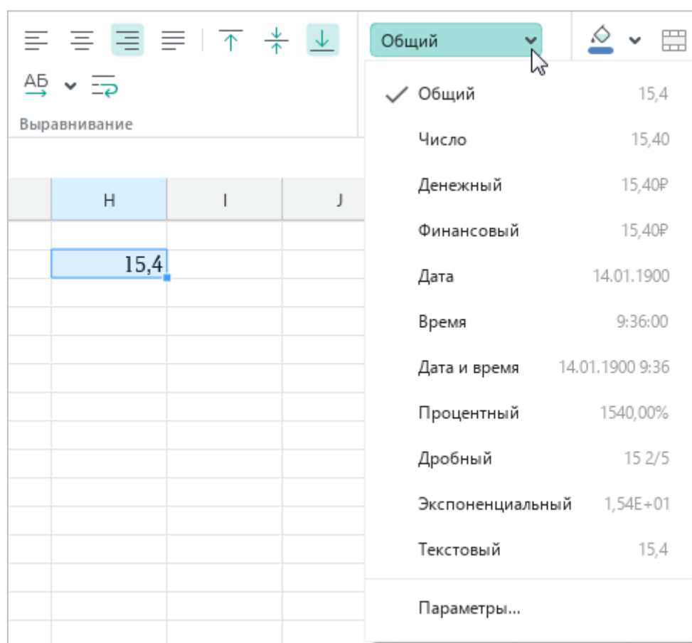
Рисунок 166 – Определение формата ячейки
