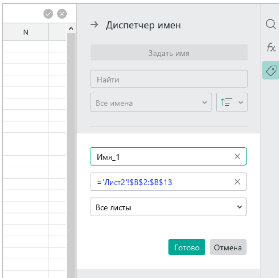
Рисунок 206 – Создание имени с помощью Диспетчера имен
