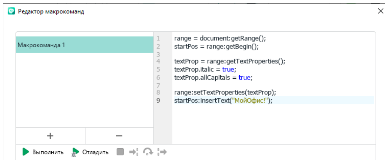
Рисунок 342 – Ввод текста макроккоманды
