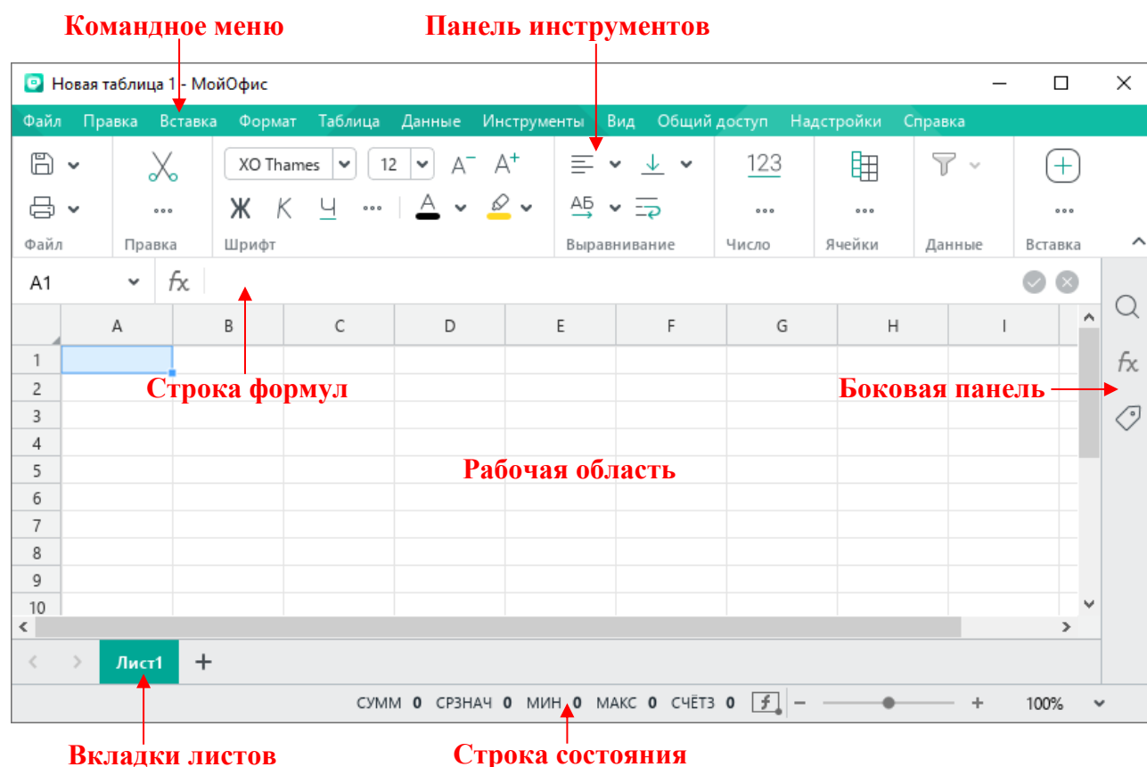
Рисунок 5 – Главное окно приложения «МойОфис Таблица»
