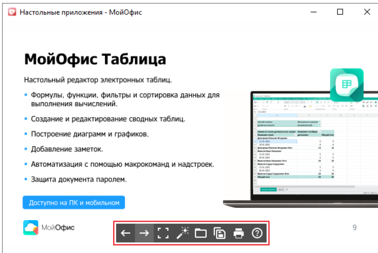
Рисунок 4 – Панель инструментов
